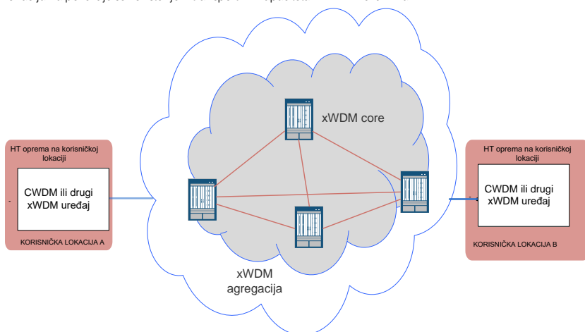
Slika 2. Načelan prikaz E2E realizacije xWDM voda
